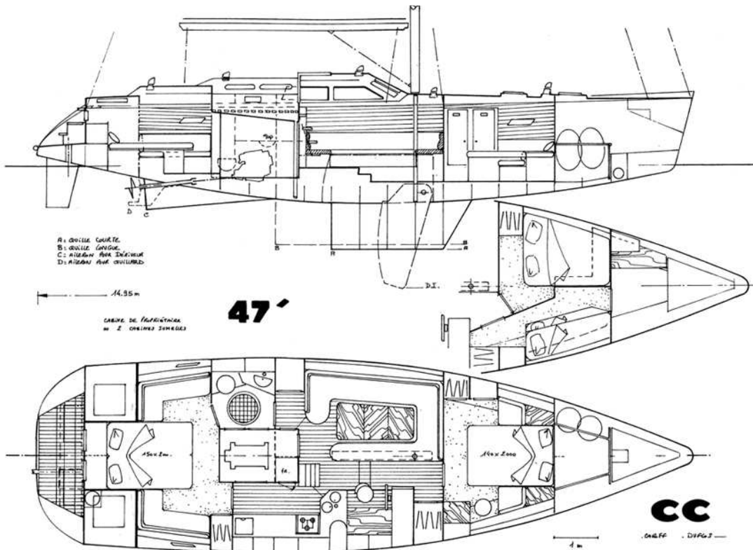
Chatam 47. Cockpit central. DI ou quillard. Cabine ou carré arrière.
