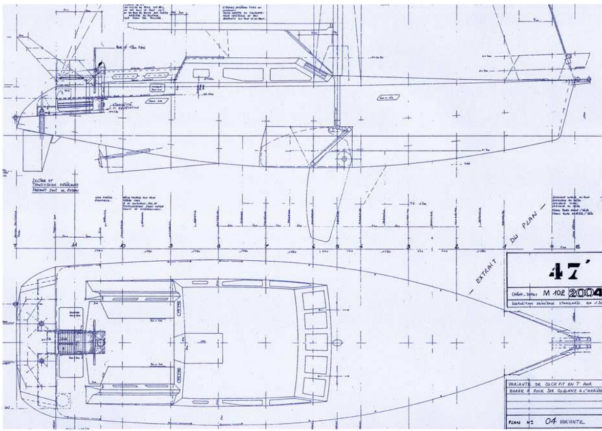
Chatam 47, DI, à salon de pont.
