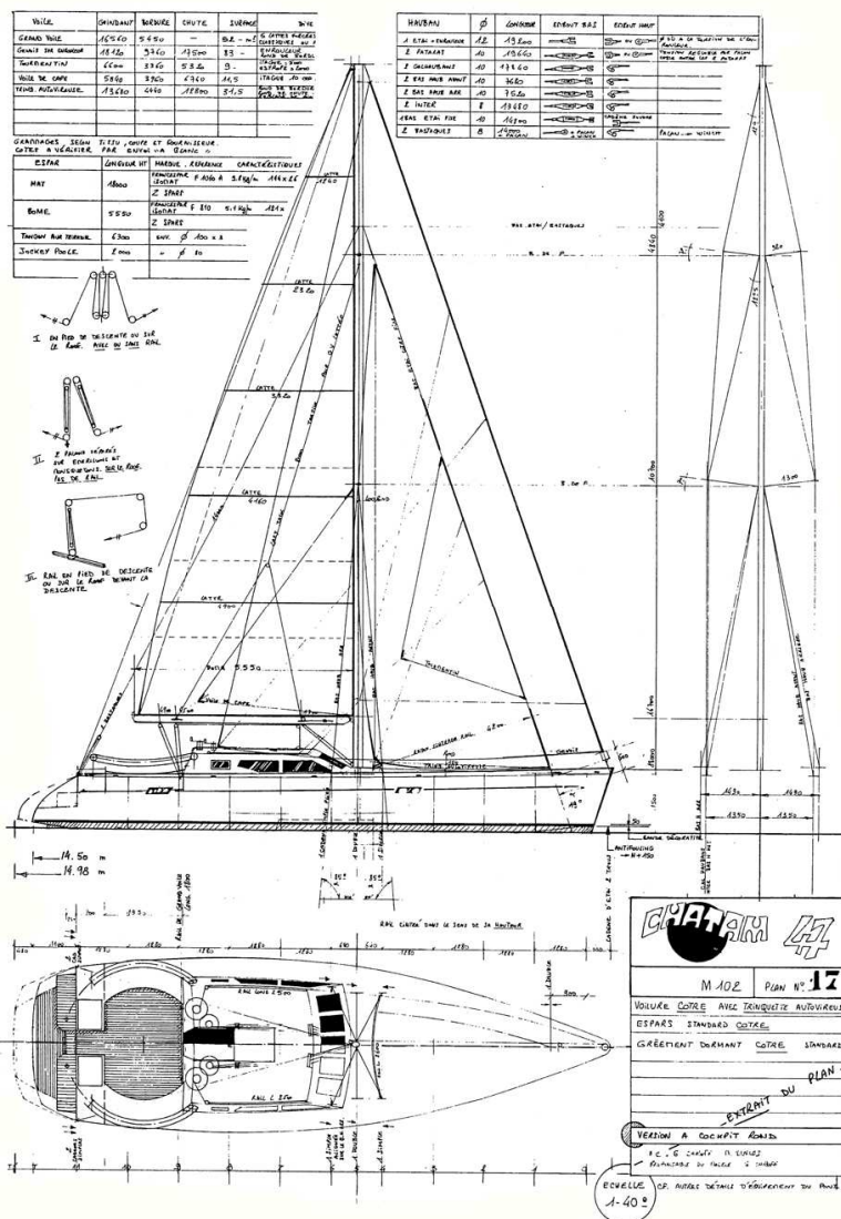
Extrait de plan de voile cotre
