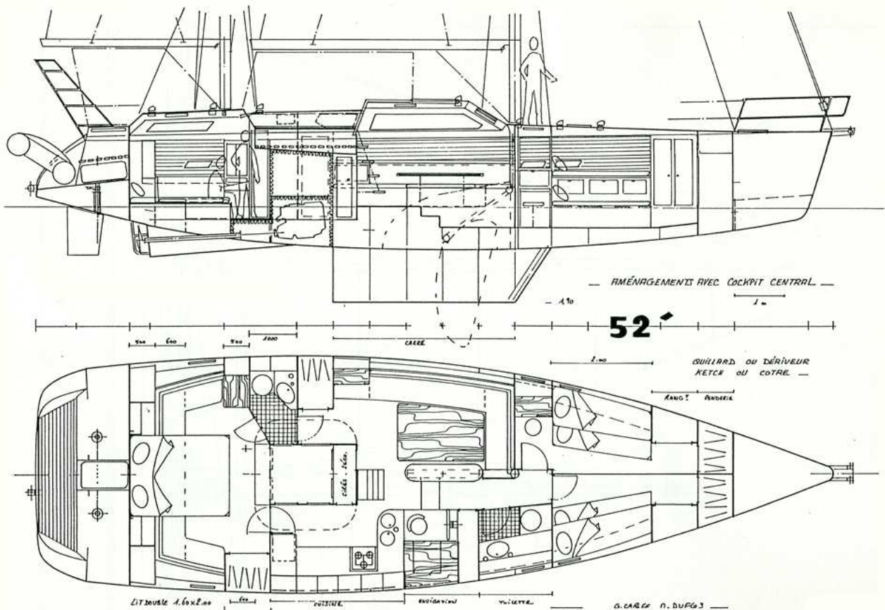
Version à cockpit central.
