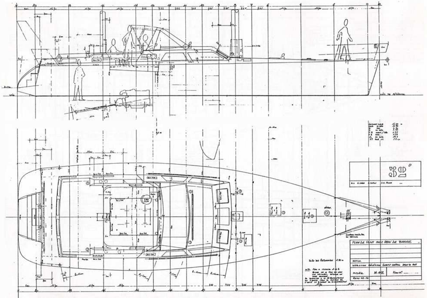
Version à cockpit central.
